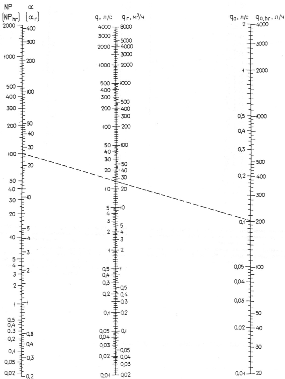
Черт. 4. Номограмма для определения секундных и часовых расходов воды в зависимости от NP ( NP_{hr} ) при различных значениях q(0) , л/с, и q(0, \text{hr}) , л/ч
